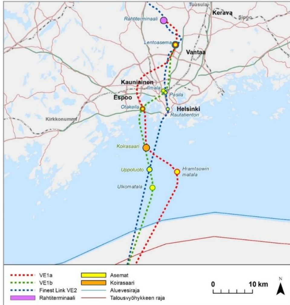
Kuva 13. Tallinna-tunnelin vaihtoehtoiset linjaukset (FinEst Bay Area 2018).
