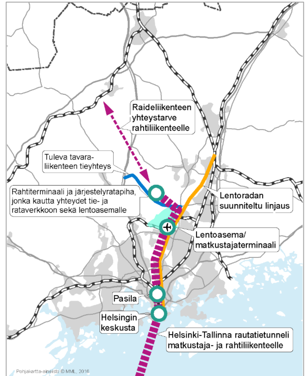
Kuva 14. Tallinna-tunnelin liittyminen liikennejärjestelmään (FinEst Link 2018).
